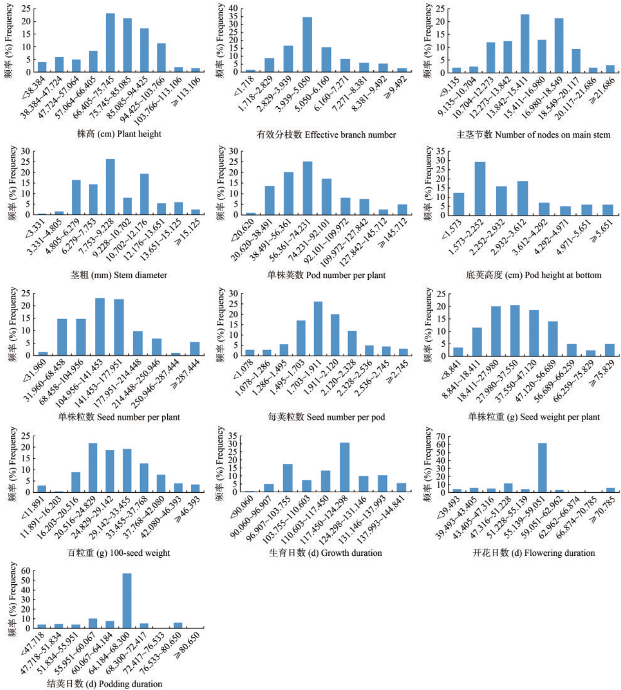
图2 数量性状的频率分布直方图
