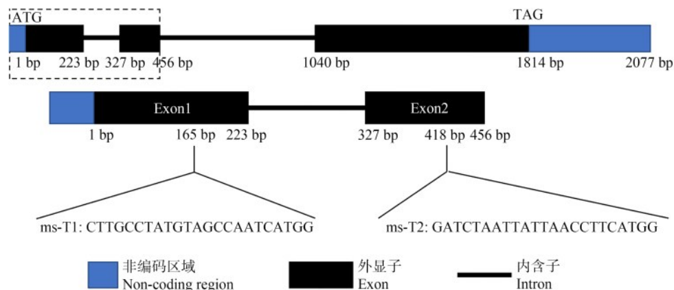
图 1 MS6 基因结构及靶点位置
