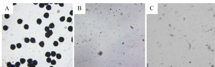
A: 野生型植株; B: T 1 代无花粉型植株; C: 用于基因定位的ms6突变体 A: Wild type plants; B: T 1 pollen-free plants; C: ms6 mutant for gene mapping
