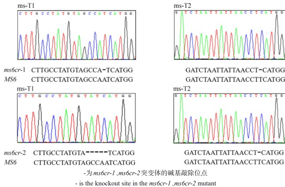
图4 T 1 代突变植株碱基突变位点
