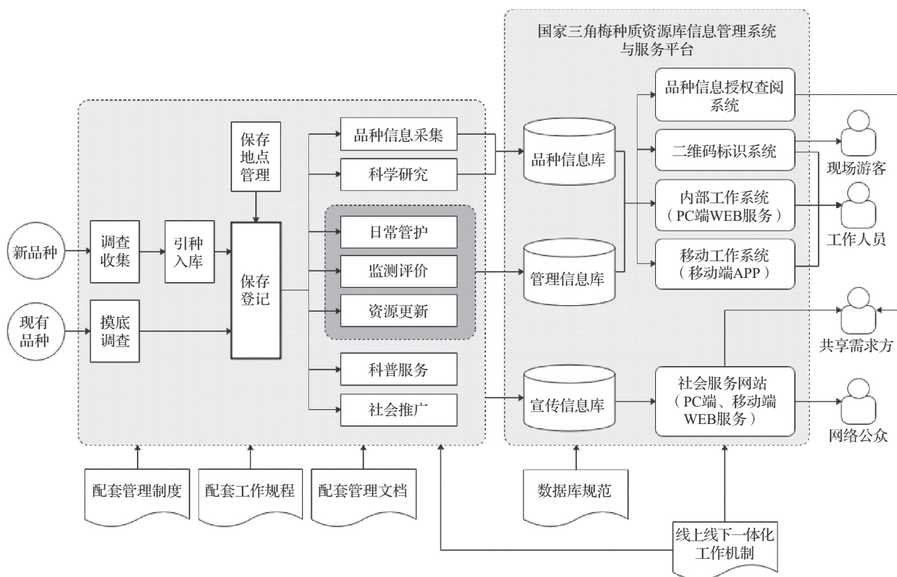
图1 平台架构
