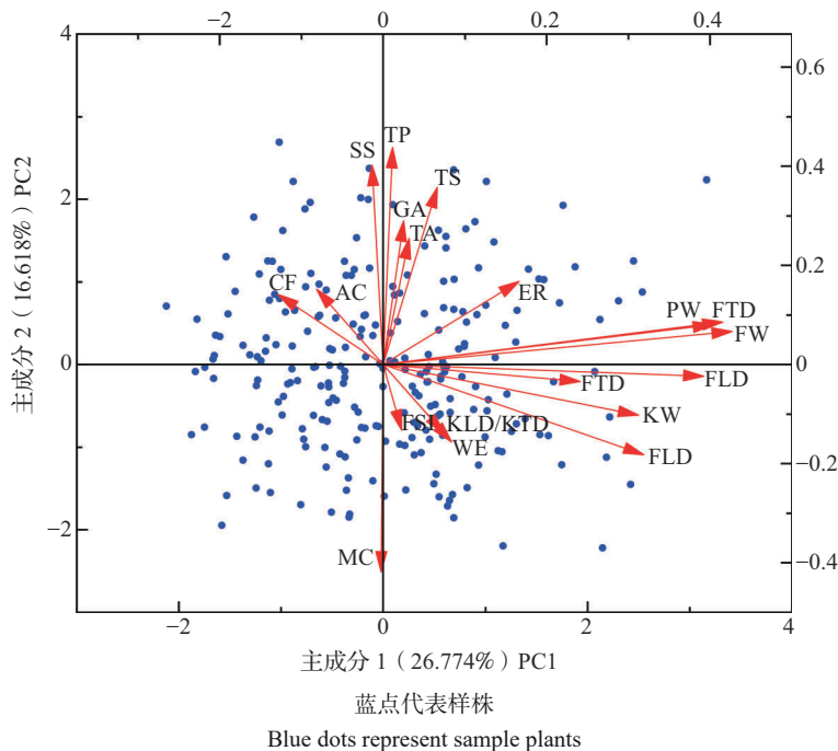
图3 诃子19个性状主成分分析
